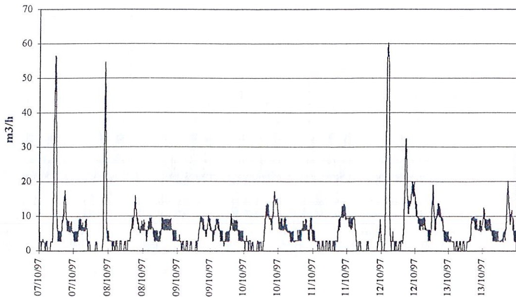
Débits sur PR5-Maillot (m3/h) du 07/10/97 au 13/10/97
